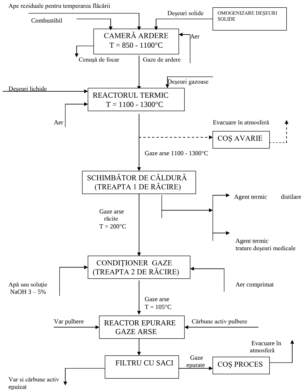
Figura 1. SCHEMA TEHNOLOGICĂ A INSTALAȚIEI DE INCINERARE DE CAPACITATE 9,8 t/ ZI
